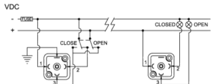
(2 CABLES) / (2 WIRES)
